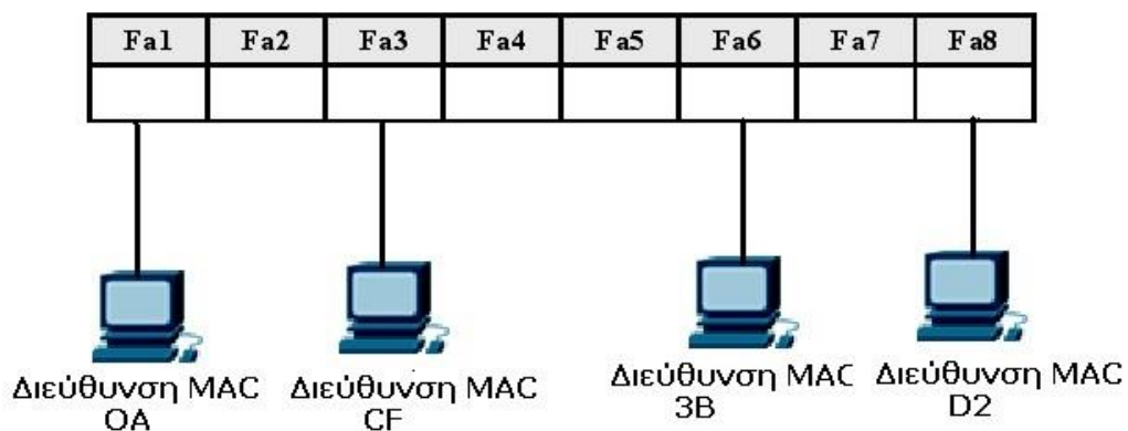
Μεταγωγέας Ethernet
