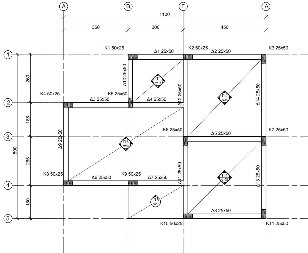
ΕΥΛΟΤΥΠΟΣ ΠΛΑΚΑΣ ΟΡΟΦΗΣ ΚΛ. 1:100
