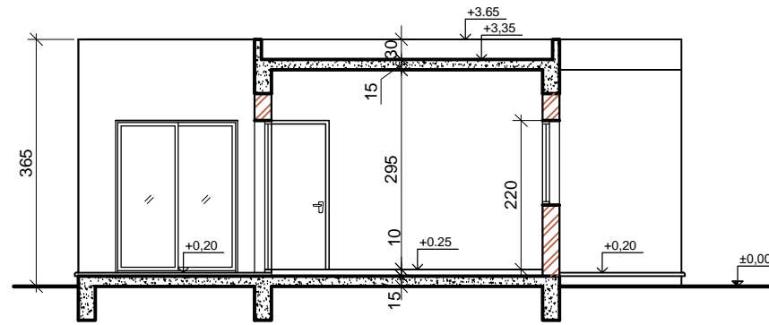
TOMH A - A ΚΛ. 1:100
