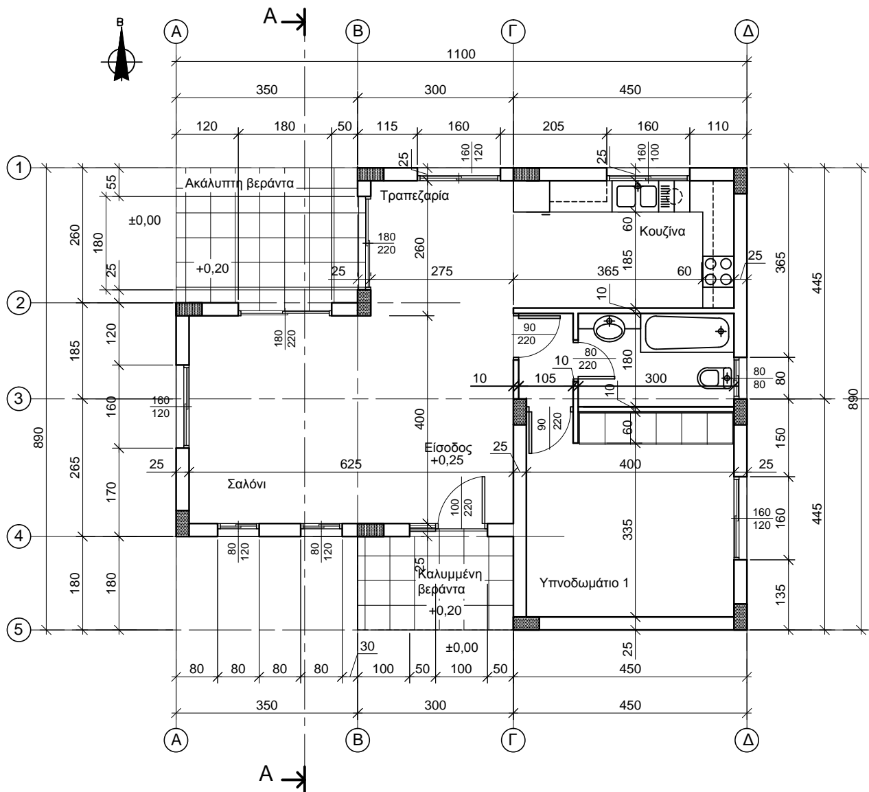
ΚΑΤΟΨΗ ΙΣΟΓΕΙΟΥ ΚΛ. 1:100
