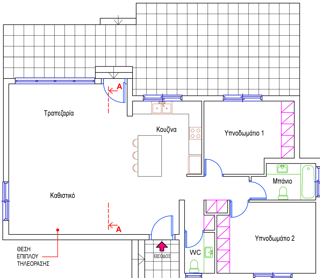
ΚΑΤΟΨΗ ΚΑΤΟΙΚΙΑΣ
