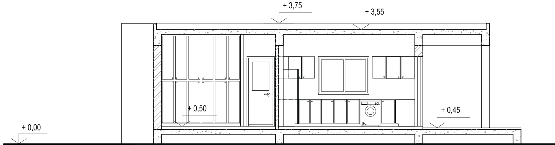
ΤΟΜΗ Β-Β
