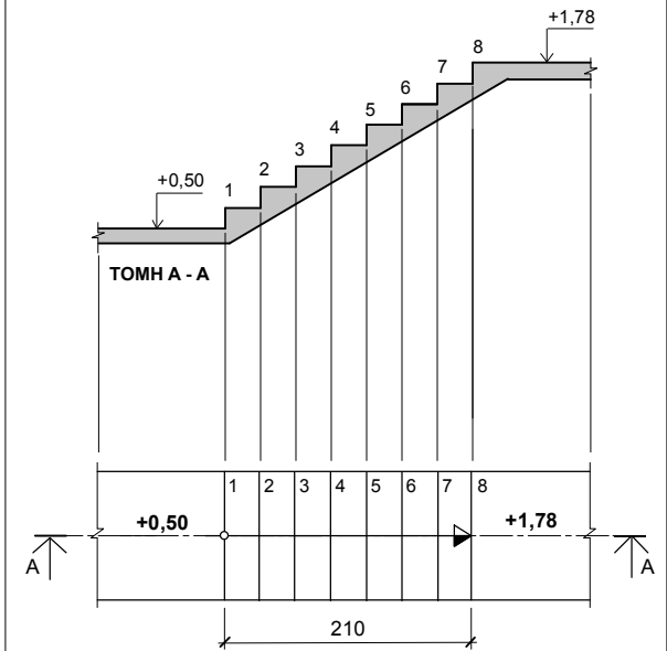
ΚΑΤΟΨΗ ΚΛ. 1:50
