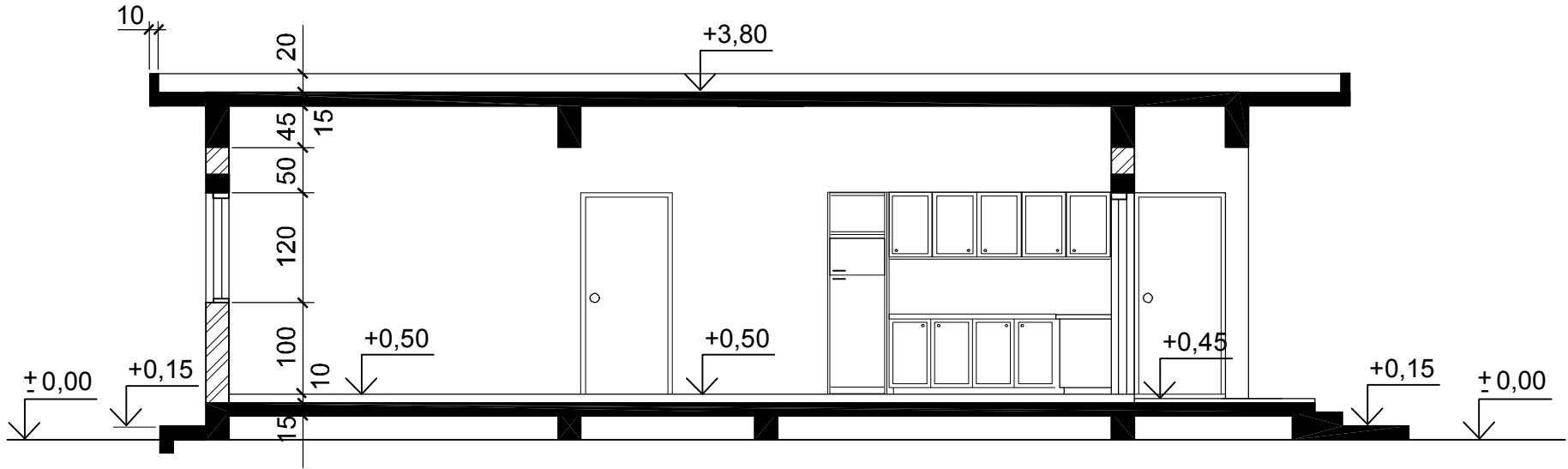
ΤΟΜΗ Α-Α ΚΛ. 1:50
