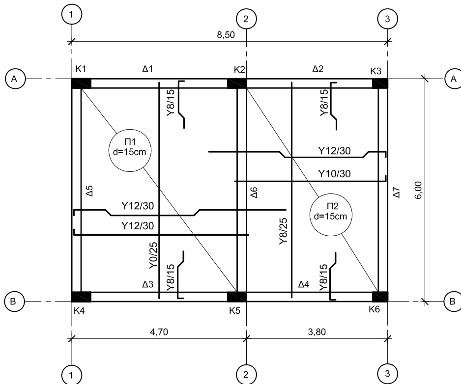
ΚΑΤΟΨΗ ΞΥΛΟΤΥΠΟΥ ΠΛΑΚΑΣ
