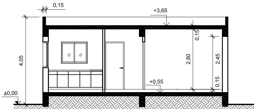
ΤΟΜΗ Α-Α
