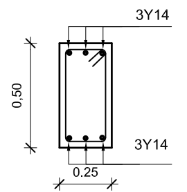
ΤΟΜΗ ΣΔ1 ΚΛ. 1:25
