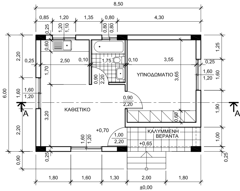
ΚΑΤΟΨΗ
