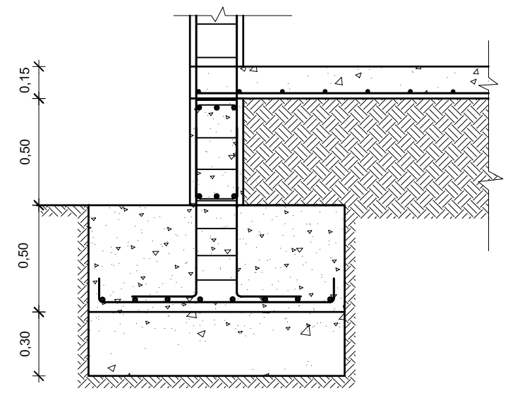
ΤΟΜΗ ΠΕΔΙΛΟΥ Κ1 ΚΛ. 1:25
