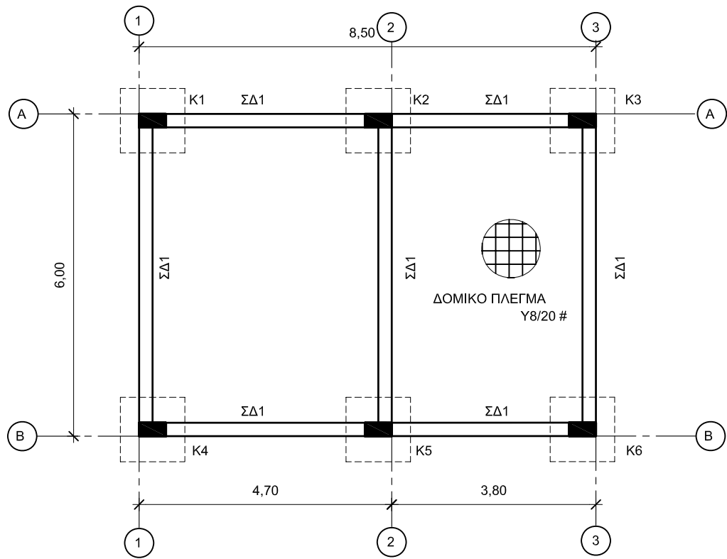
ΚΑΤΟΨΗ ΘΕΜΕΛΙΩΝ ΚΛ. 1:100
