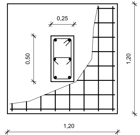
ΚΑΤΟΨΗ ΠΕΔΙΛΟΥ Κ1 ΚΛ. 1:25
