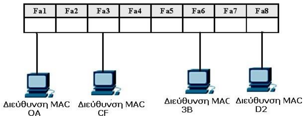
Μεταγωγέας Ethernet
