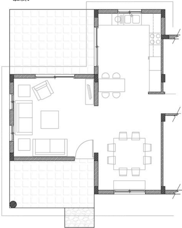
ΚΑΤΩΦΗ ΚΛΙΜΑΚΑ 1:50
