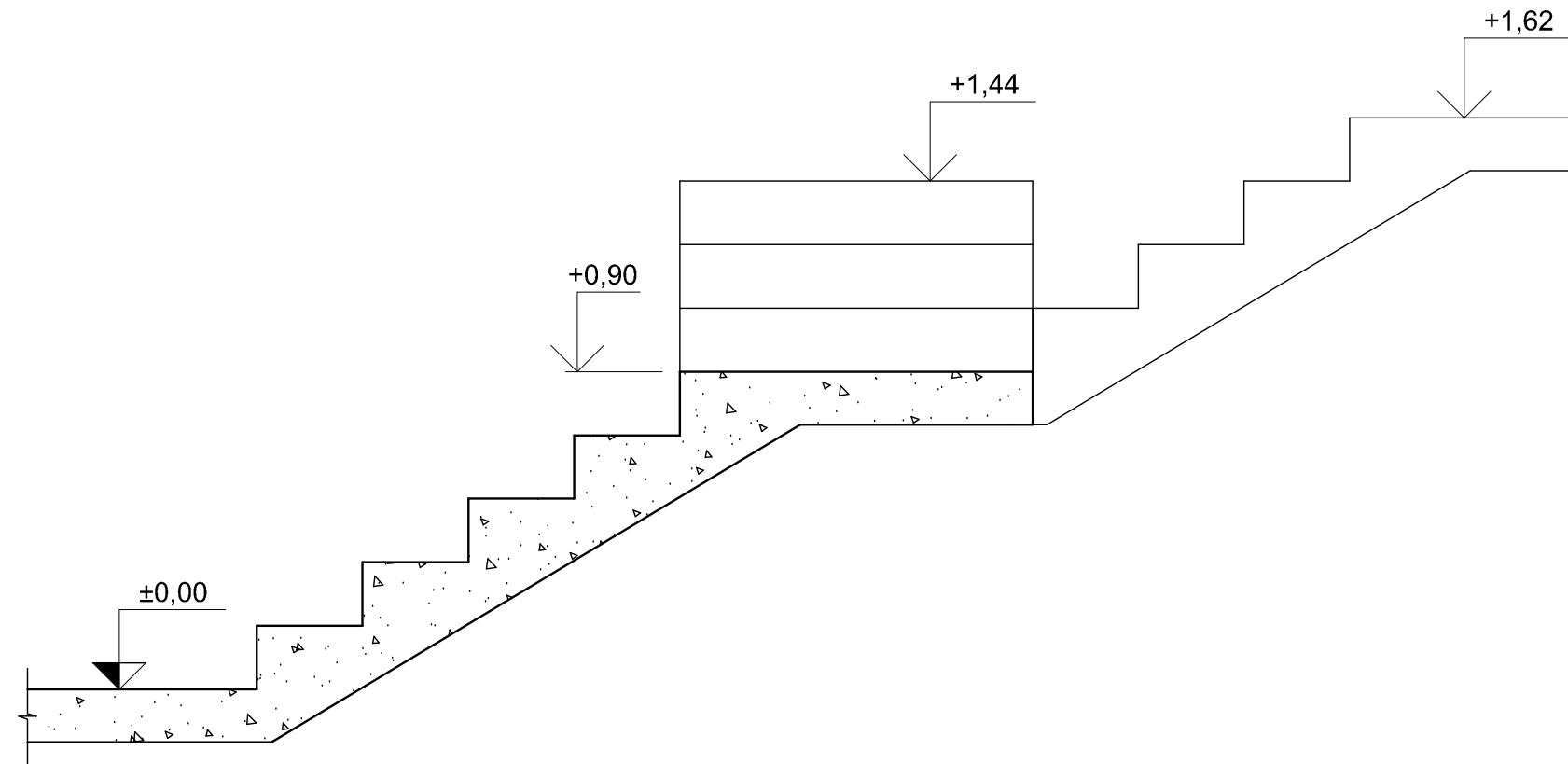
ΤΟΜΗ 1-1 ΣΚΑΛΑΣ ΚΛ. 1:20
